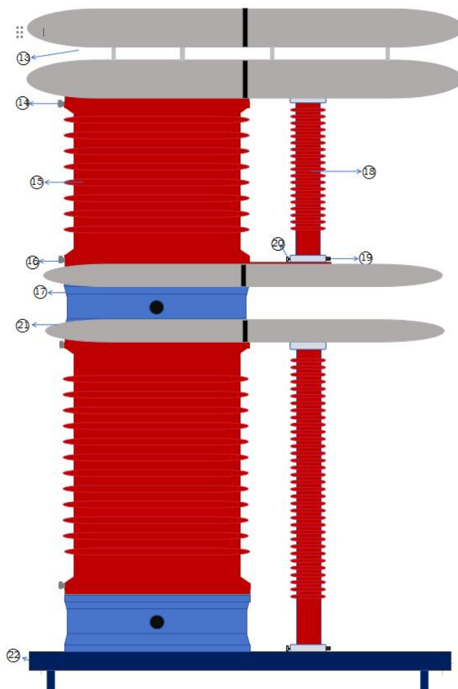
图 3 电抗器及分压器示意图
