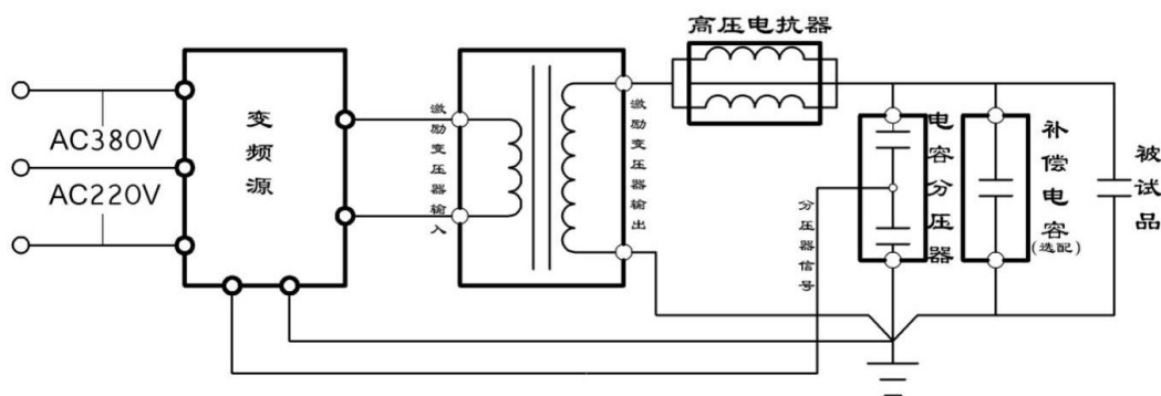
变频串联谐振试验接线图
