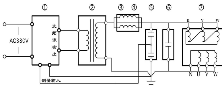
变压器耐压试验接线图
