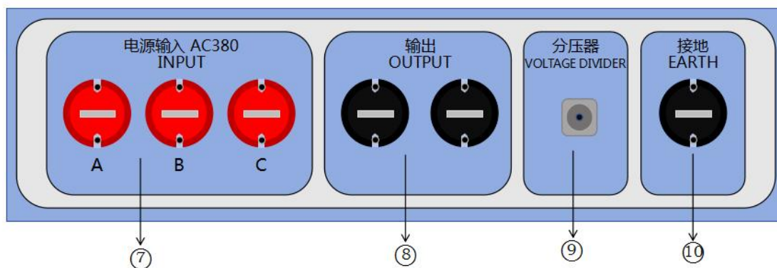
图 2 接线面板
